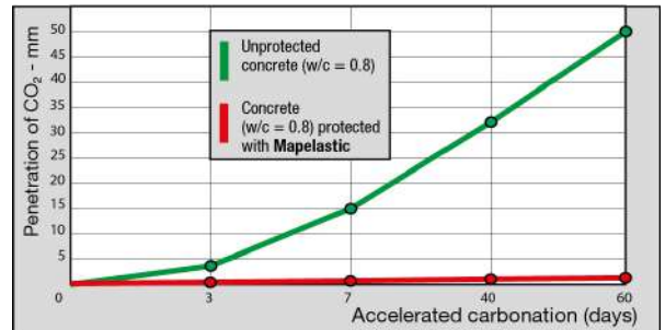
Fig. 2: Effetto di Mapelastic sulla carbonatazione accelerata (30% of CO 2 ) in un calcestruzzo poroso
